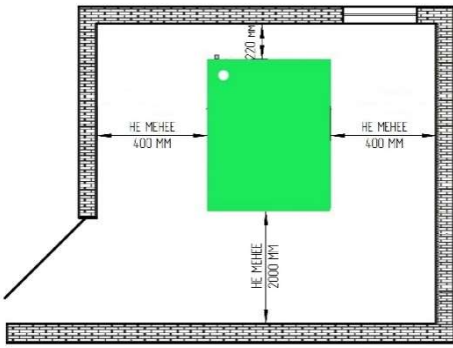
Рис. 5. Установка котла в помещении
