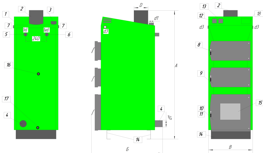
Рисунок 3. Основные размеры котлов Bioten (SL/SLE)
